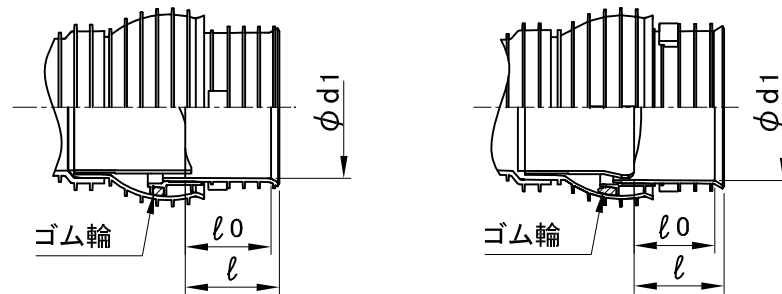
縦断面図
