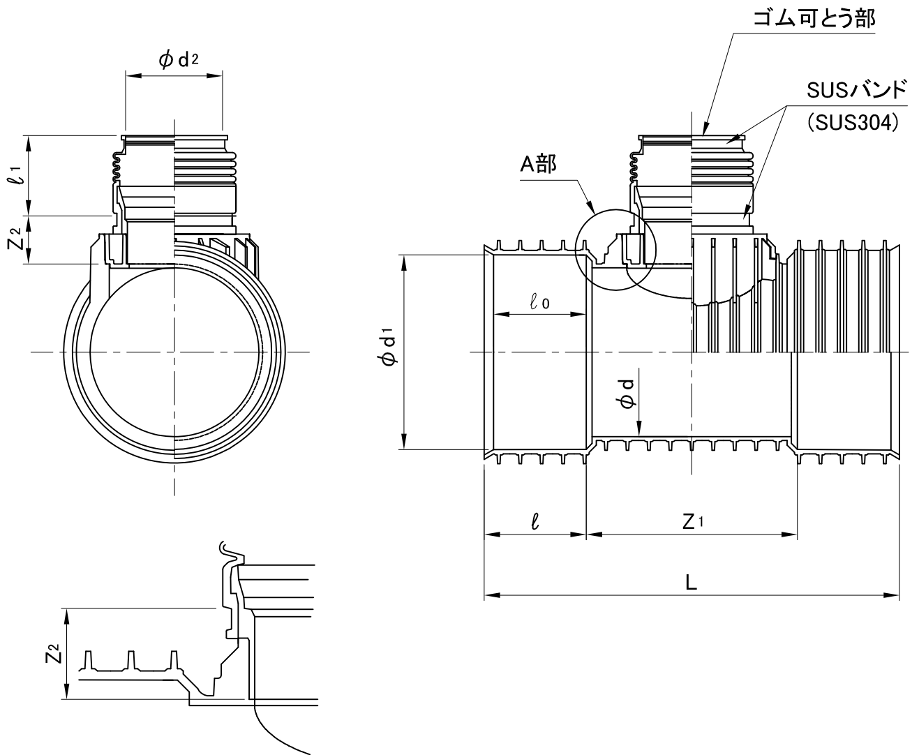
呼び径 150-100 および 200-150A部の形状
