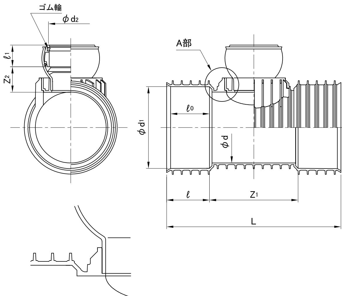
呼び径150-100、150-125および200-150 A部の形状
