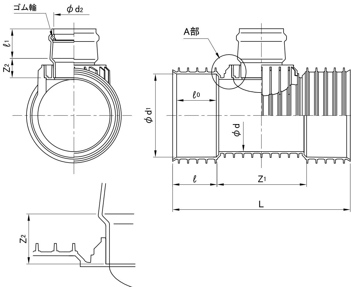
呼び径 150-100、150-125および200-150 A部の形状
