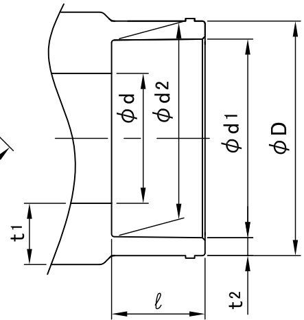
接合部寸法
