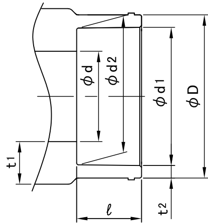
接合部寸法
