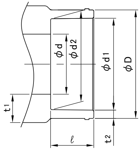
接合部寸法
