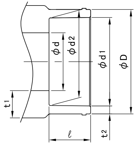
接合部寸法
