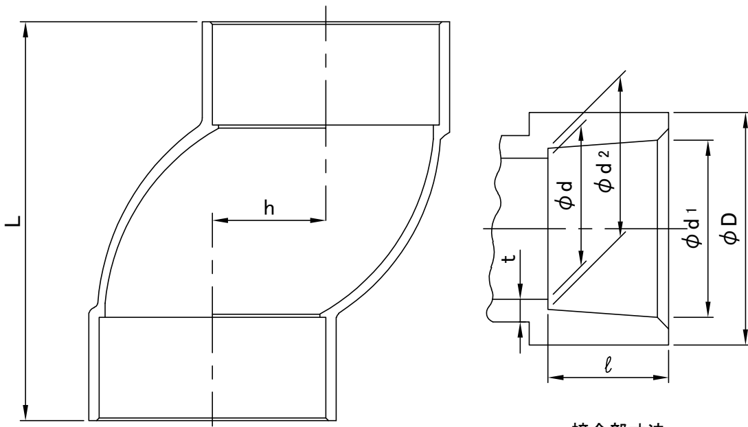
接合部寸法
