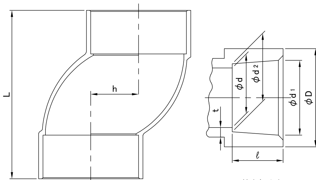
接合部寸法
