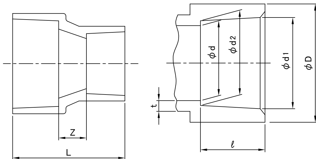
接合部寸法
