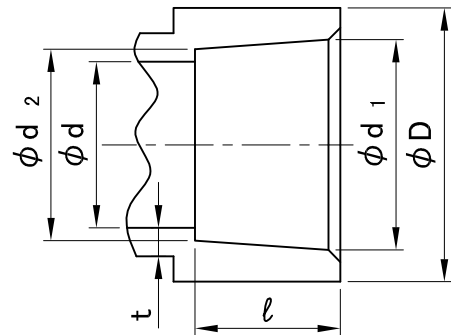
接合部共通図
