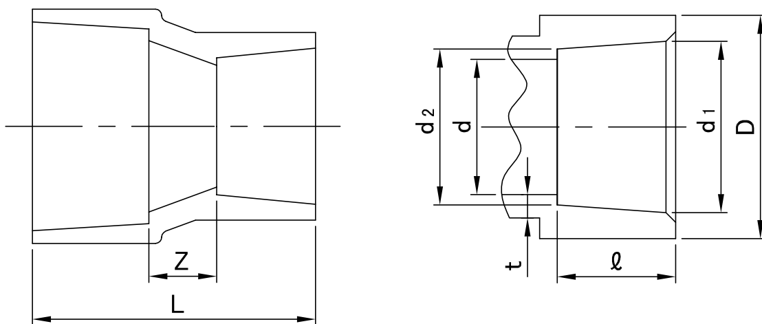
接合部寸法
