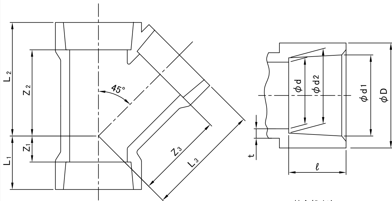
接合部寸法
