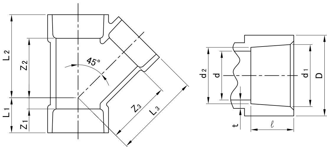
接合部共通図
