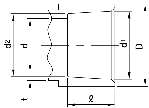
接合部寸法
