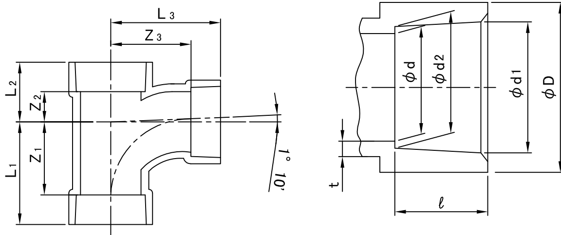
接合部寸法
