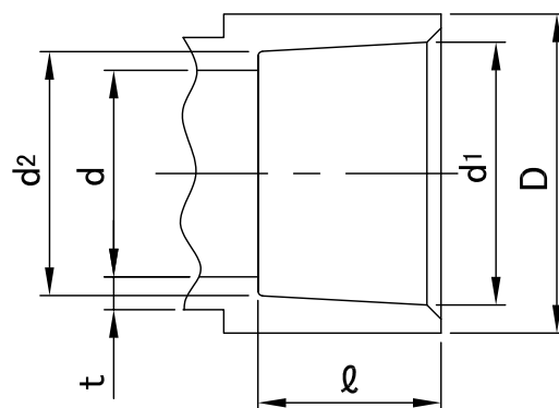
接合部寸法
