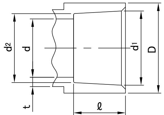
接合部寸法
