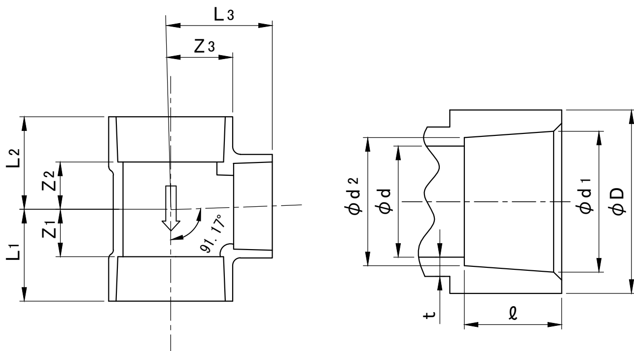
接合部寸法
