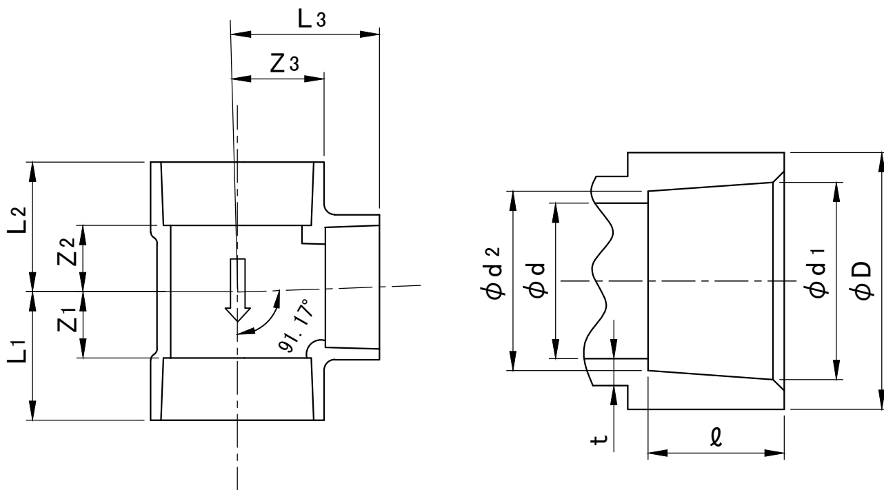
接合部寸法
