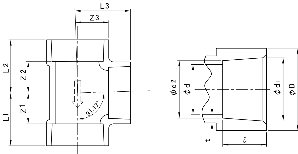
接合部寸法
