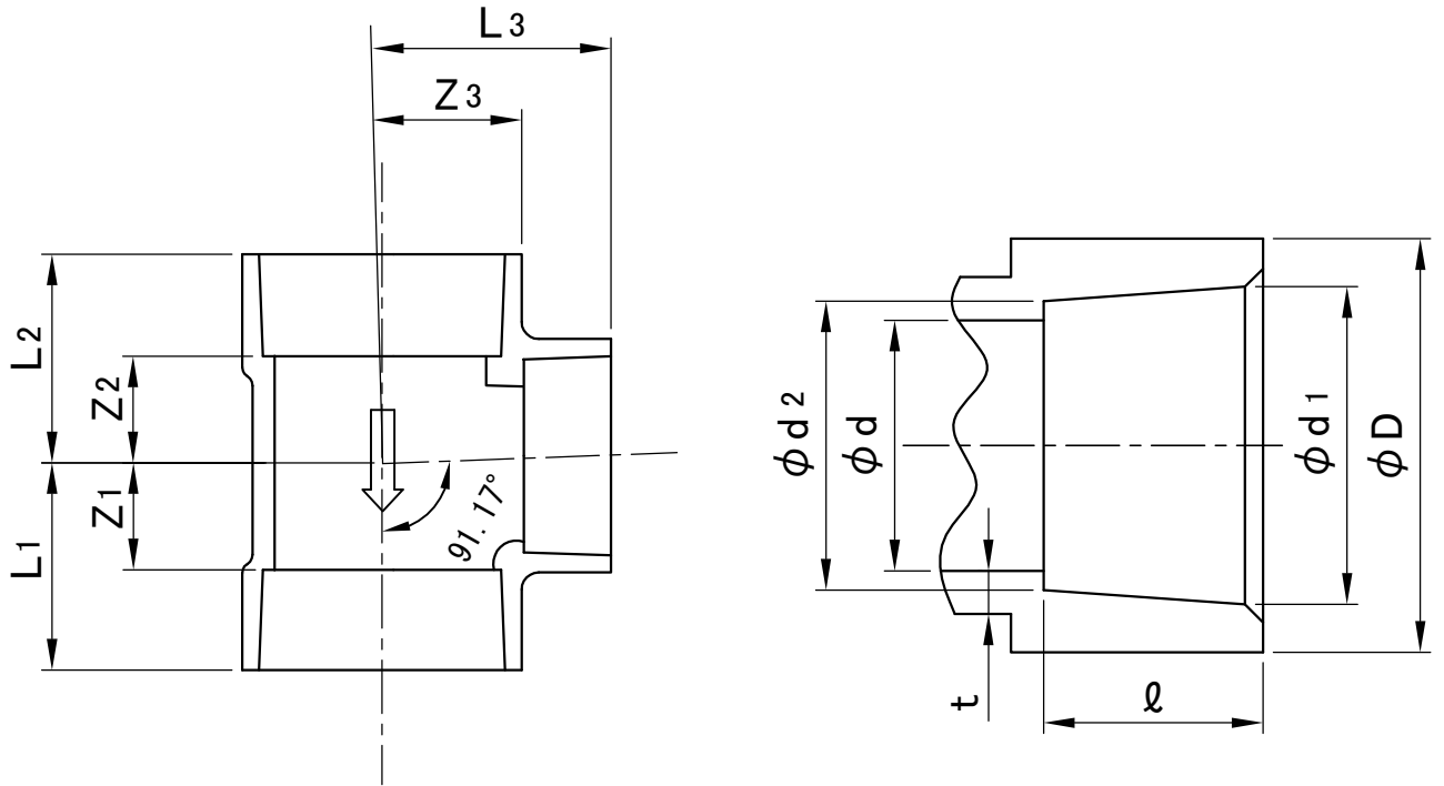
接合部寸法
