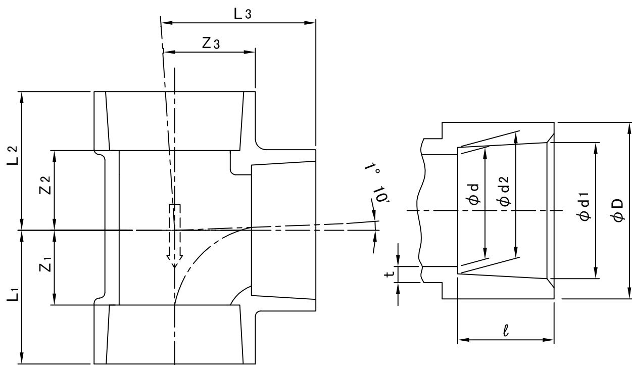
接合部寸法
