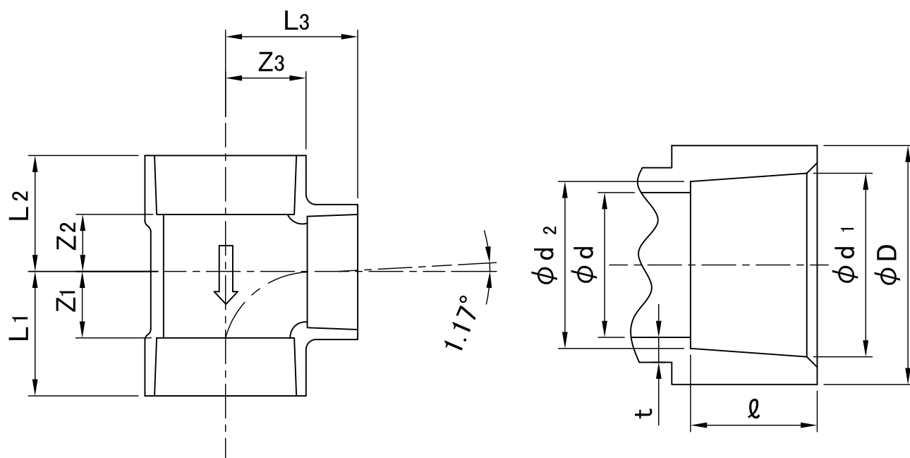
接合部寸法
