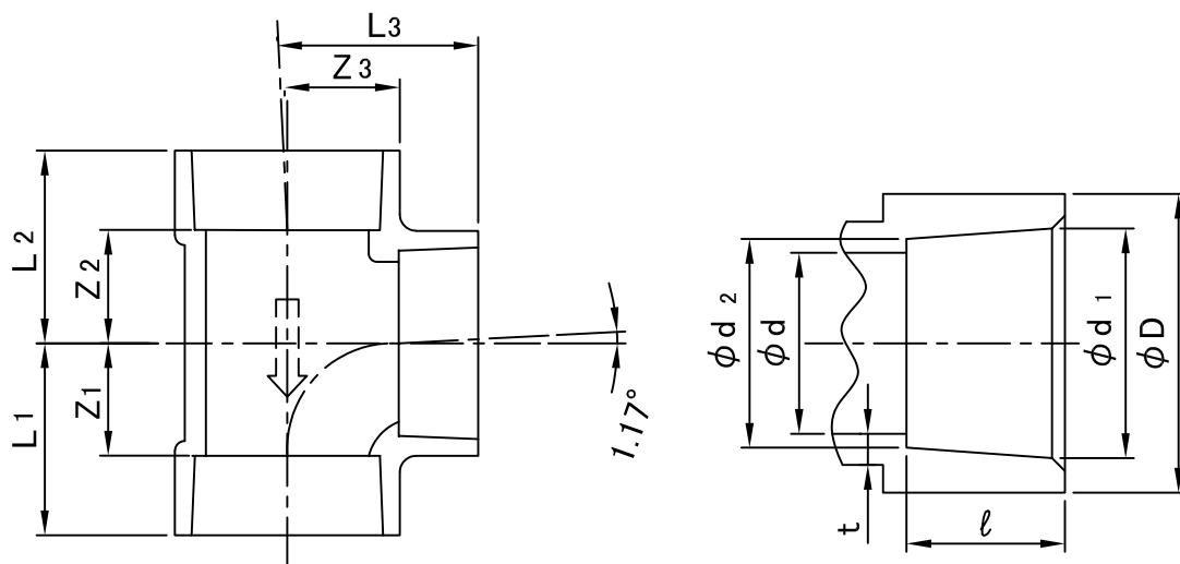
接合部寸法
