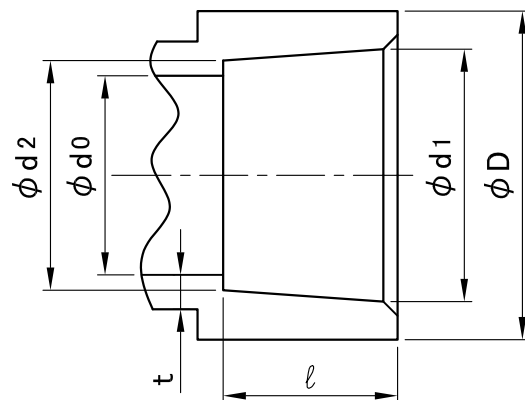
接合部寸法
