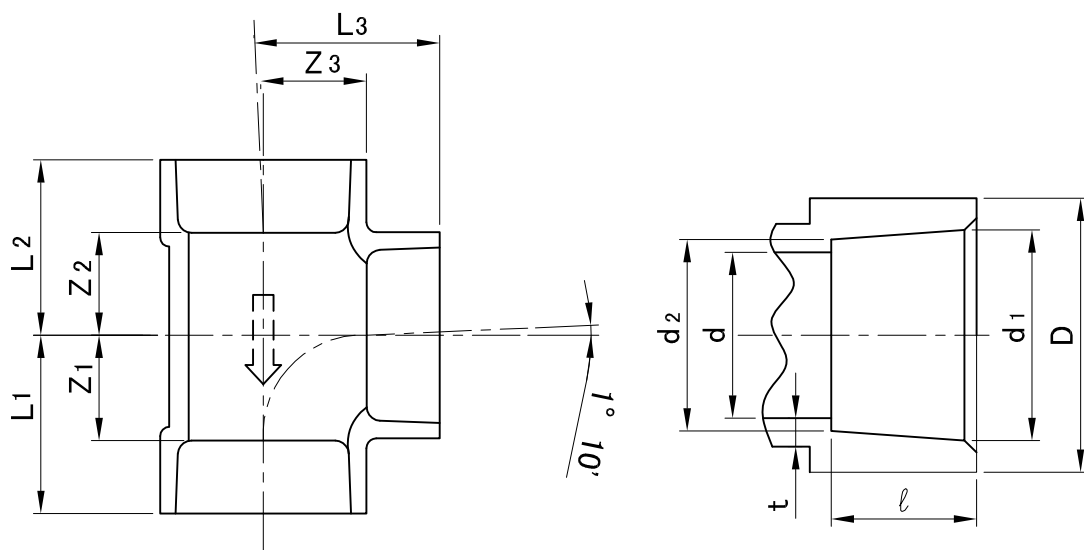
接合部共通図
