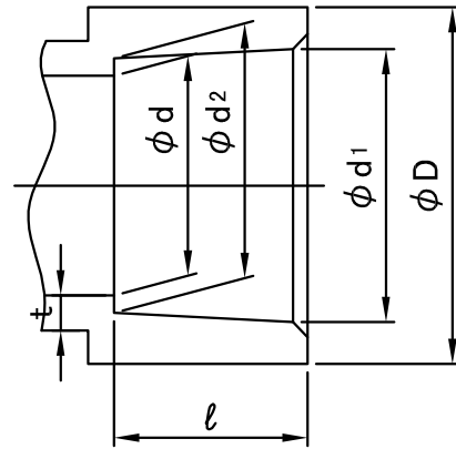
接合部寸法
