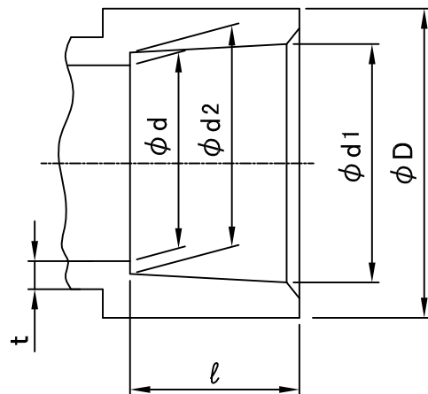
接合部寸法
