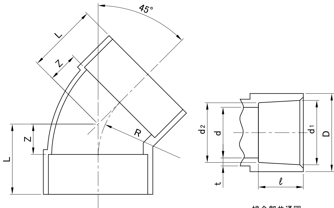
接合部共通図
