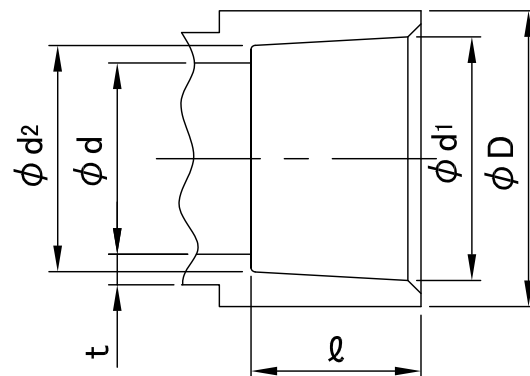
接合部共通図
