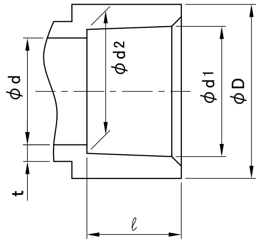
接合部寸法
