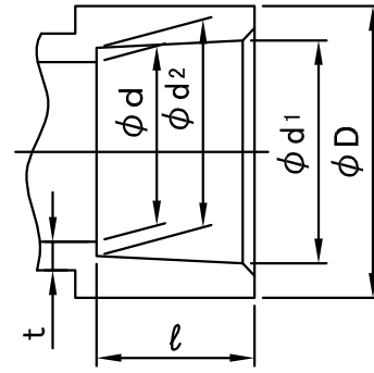
接合部寸法
