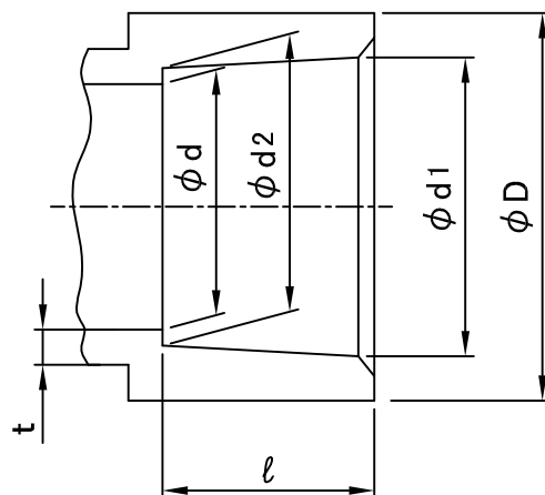
接合部寸法
