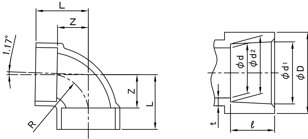
接合部寸法
