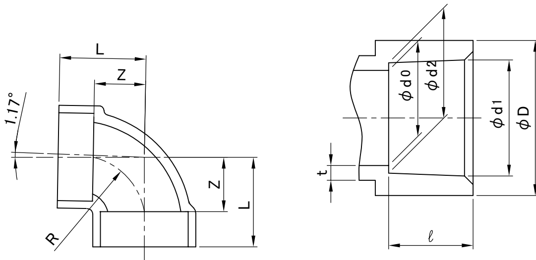
接合部寸法
