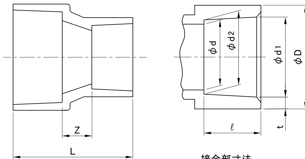
接合部寸法
