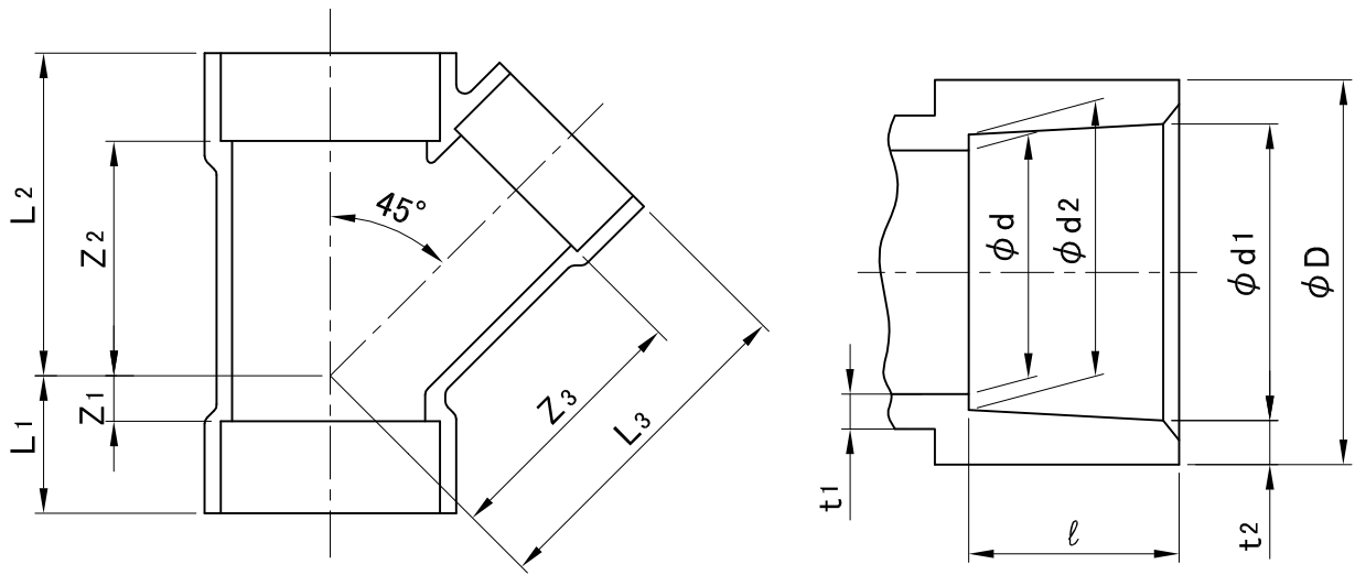
接合部寸法
