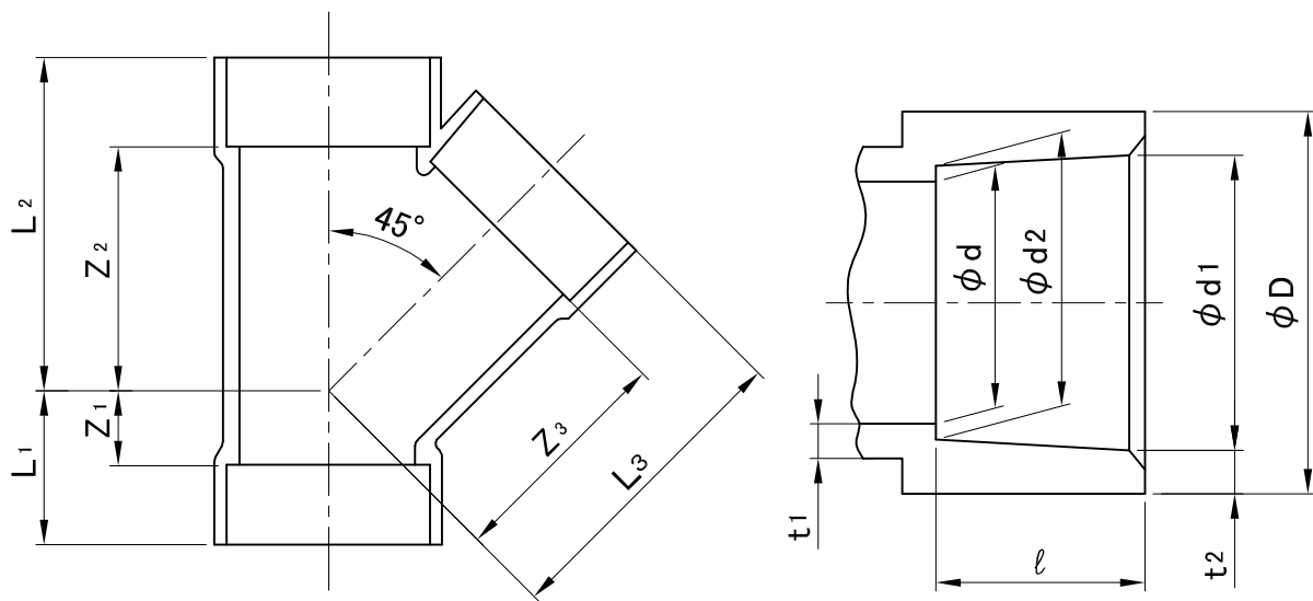
接合部寸法
