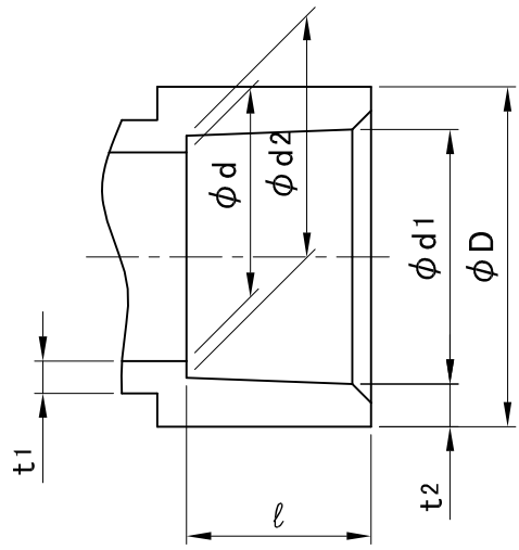
接合部寸法
