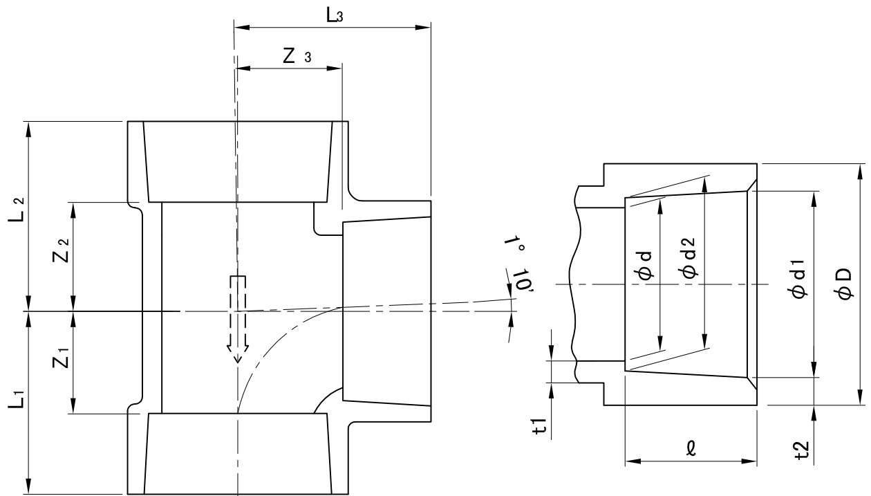
接合部寸法
