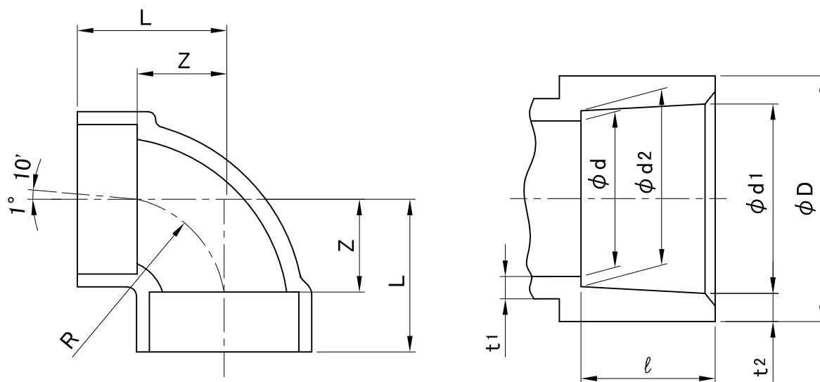
接合部寸法
