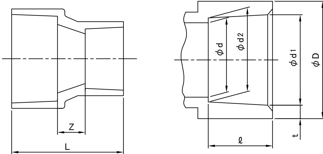
接合部寸法
