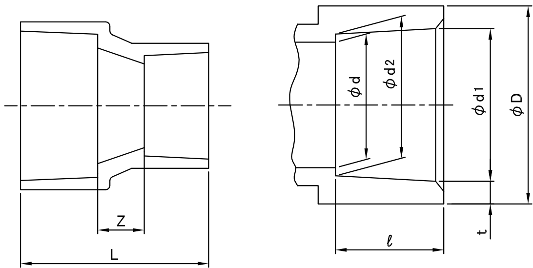
接合部寸法
