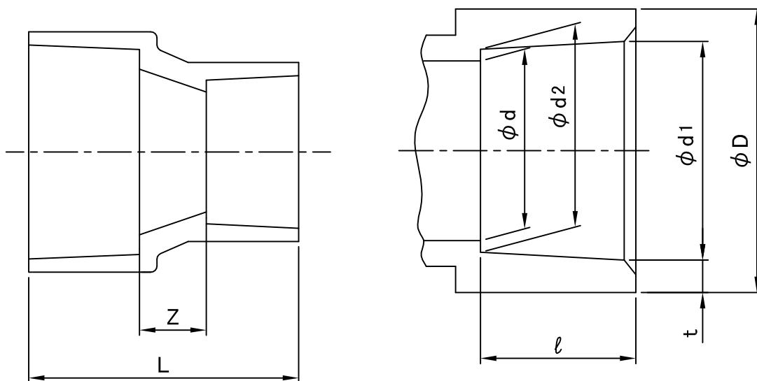
接合部寸法
