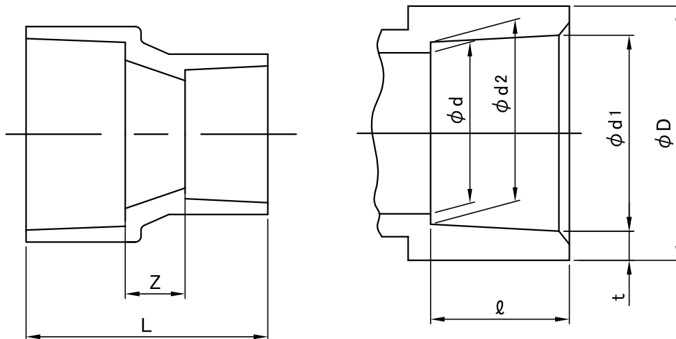
接合部寸法
