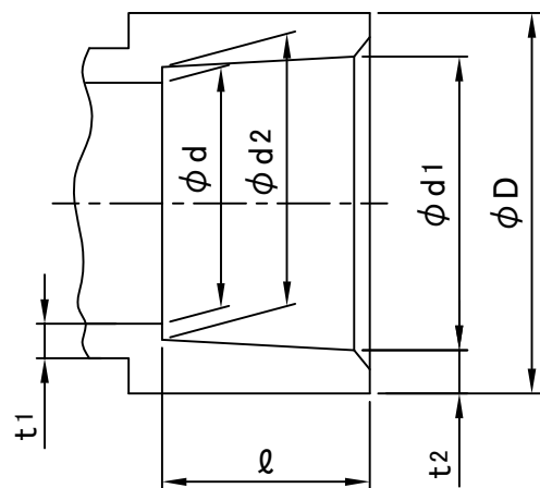
接合部寸法
