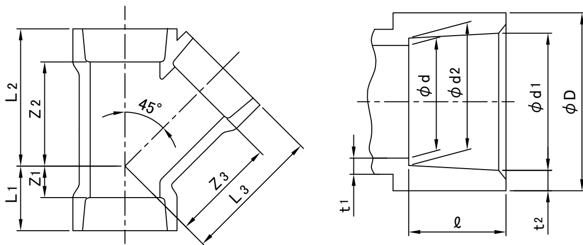
接合部寸法
