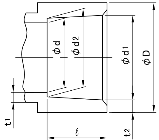
接合部寸法
